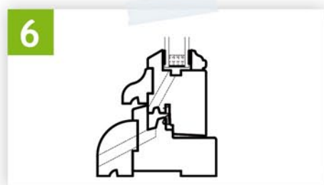
6 Nez d'appui ou seuil alu de 42 mm
